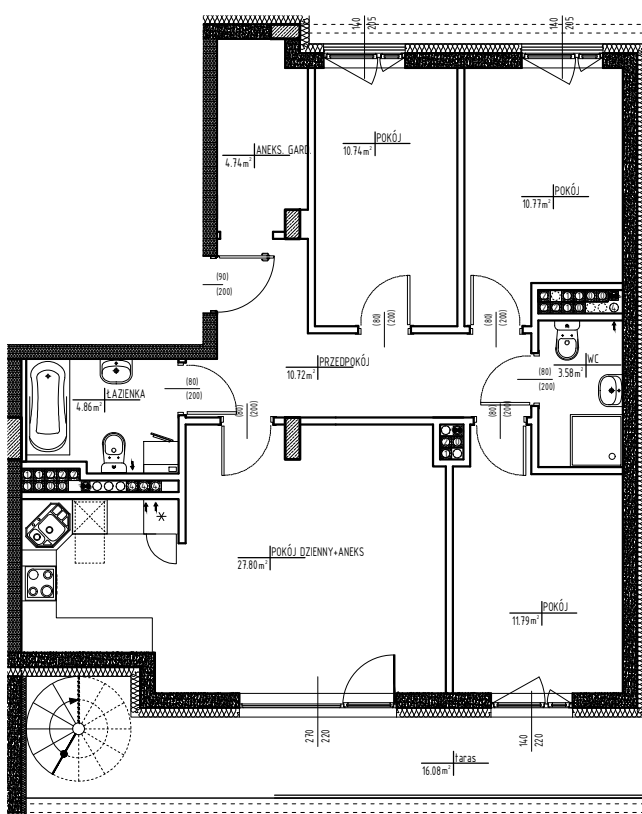
Rzut mieszkania
