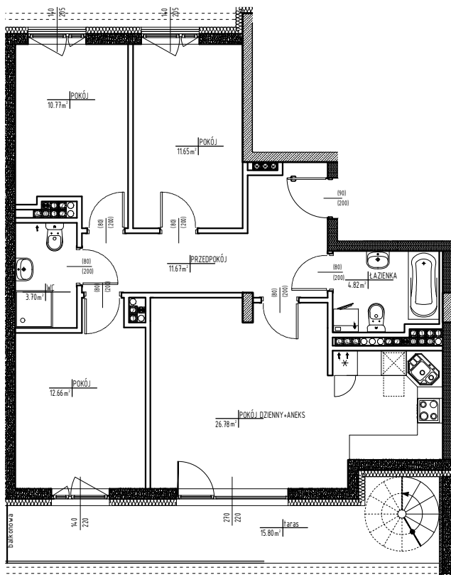
Rzut mieszkania
